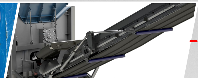
Austragsförderband 25°- 35°
